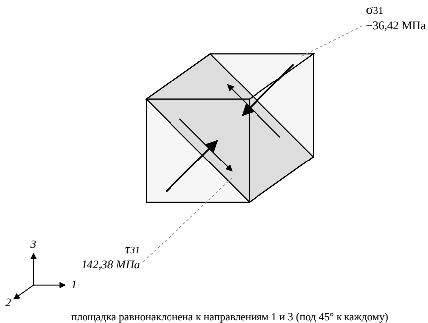
Рис. 1.3 — диагональная площадка, равнонаклонённая к главным направлениям 1 и 3: наибольшее касательное \tau_{31} = 142,38 МПа и нормальное \sigma_{31} = -36,42 МПа.
