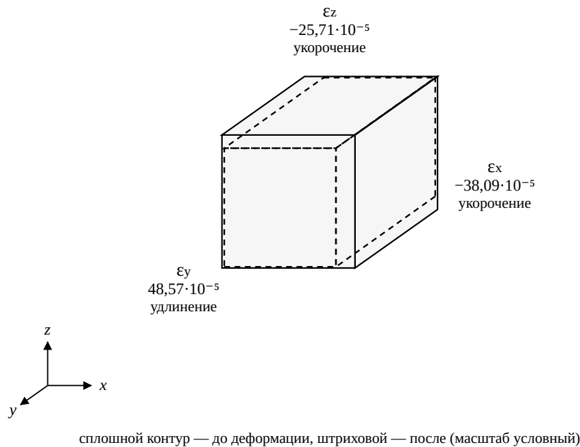
Рис. 1.4 — относительные линейные деформации: сплошной контур — до деформации, штриховой — после (масштаб условный).
