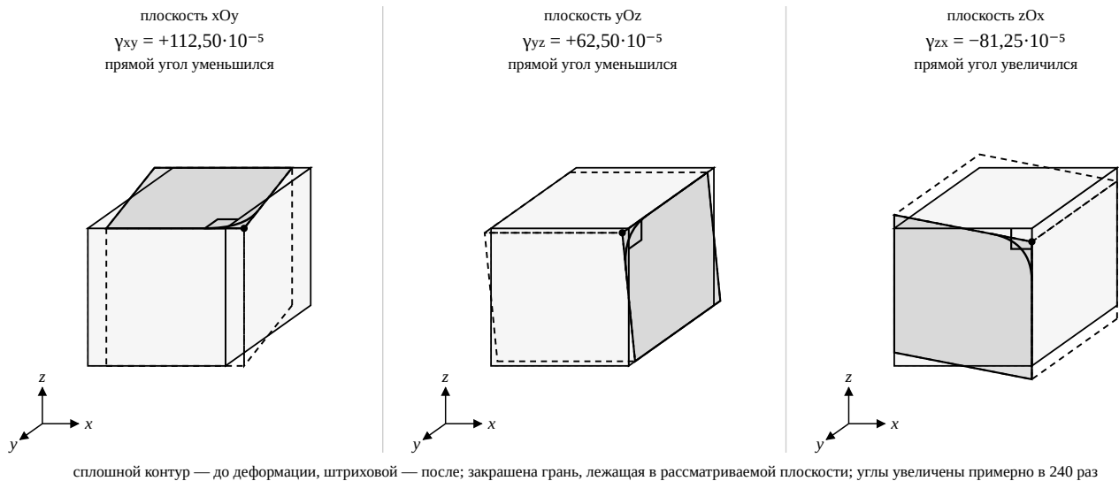
Рис. 1.5 — относительные угловые деформации: три элемента, на каждом показан сдвиг в своей координатной плоскости. Закрашена грань, лежащая в этой плоскости; у ближней вершины отмечены исходный прямой угол и угол после деформации. Сплошной контур — до деформации, штриховой — после; углы увеличены примерно в 240 раз (масштаб условный).
