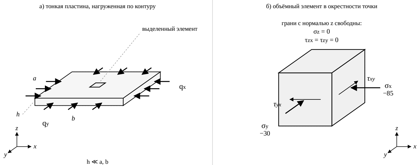
Рис. 2.1 — тонкая пластина, нагруженная по контуру (а), и выделенный из неё объёмный элемент (б): грани с нормалью z свободны от напряжений.
